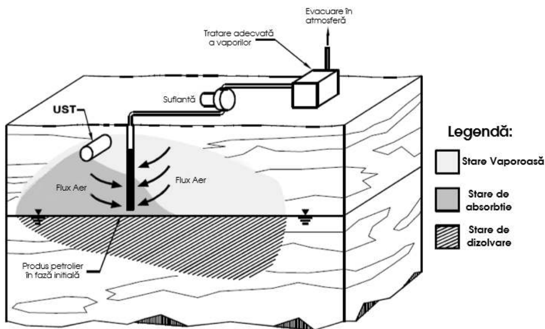
Figura 4.1- Schema cu o singură suflantă
