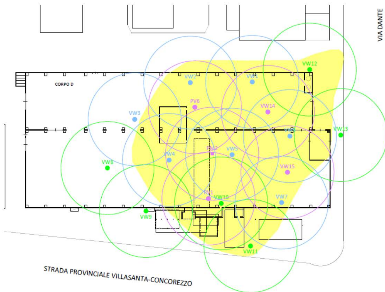
Figura 4.1- Raza de influență după Testul pilot (Confalonieri et al., see Annex1)
