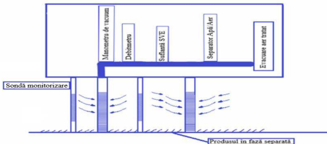
Figura 2.1- Componentele instalației SVE
