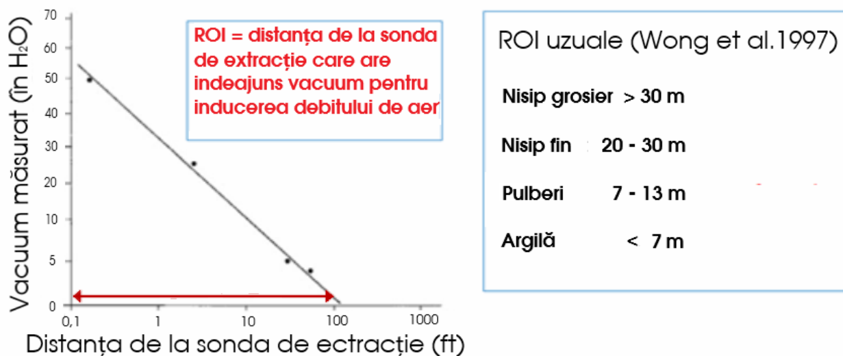
Figura 2.4- Raza de influență
