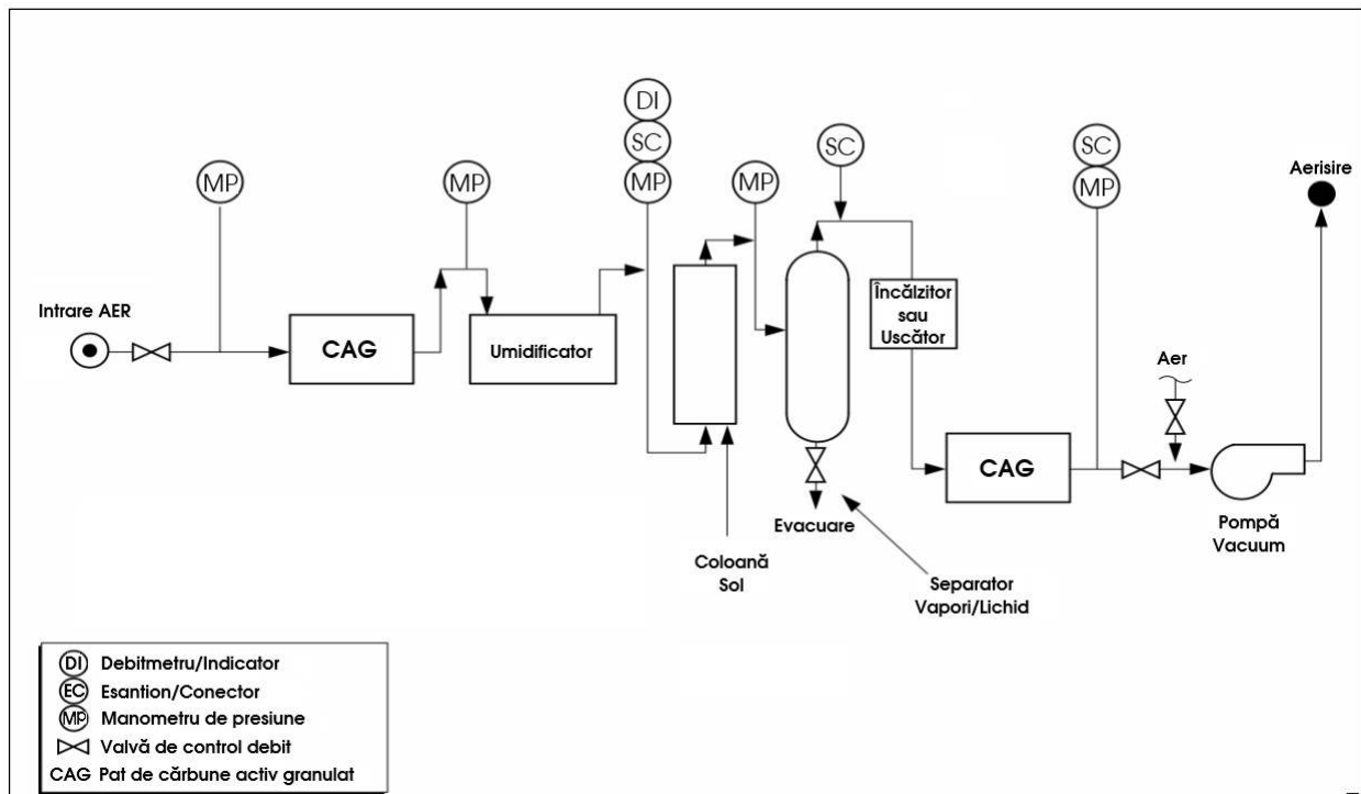
Figura 3.3- Diagrama unui aparat de testare pe coloană
