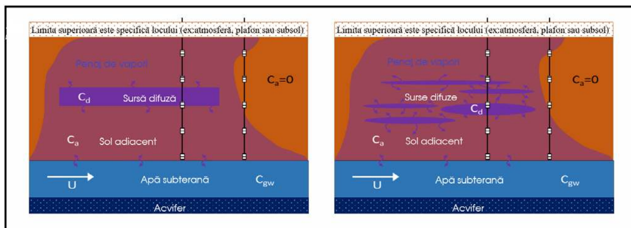
Figura 4.3- Scenarii conceptualizate pentru transferul de masă cu difuzie limitată și puncte tipice de monitorizare a gazelor din sol
