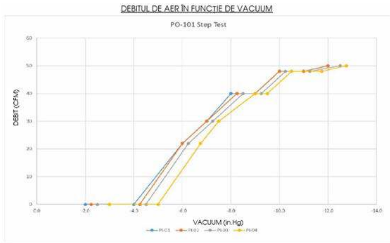
Figure 4.7- Exemplu de test de creștere a vidului în trepte SVE (Menozzi et al., vezi Anexa 1)
