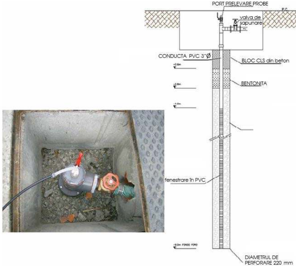
Figura 4.1- Exemplul unei instalatii Nesty (Trezzi et al., vezi Anexa 1)
