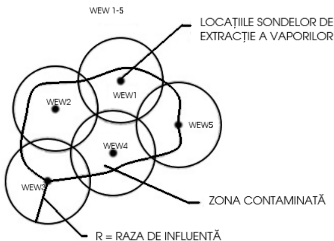
Figura 2.5- Numărul de foraje
