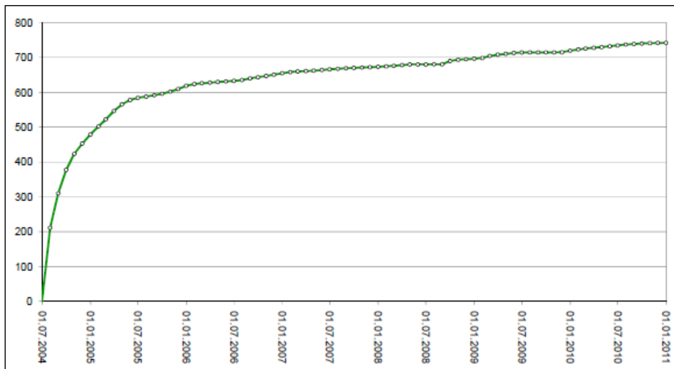
Figura 5.2 – Tendințe în eliminarea masei de contaminanți (SVE), kg PCE (total de-a lungul timpului)
