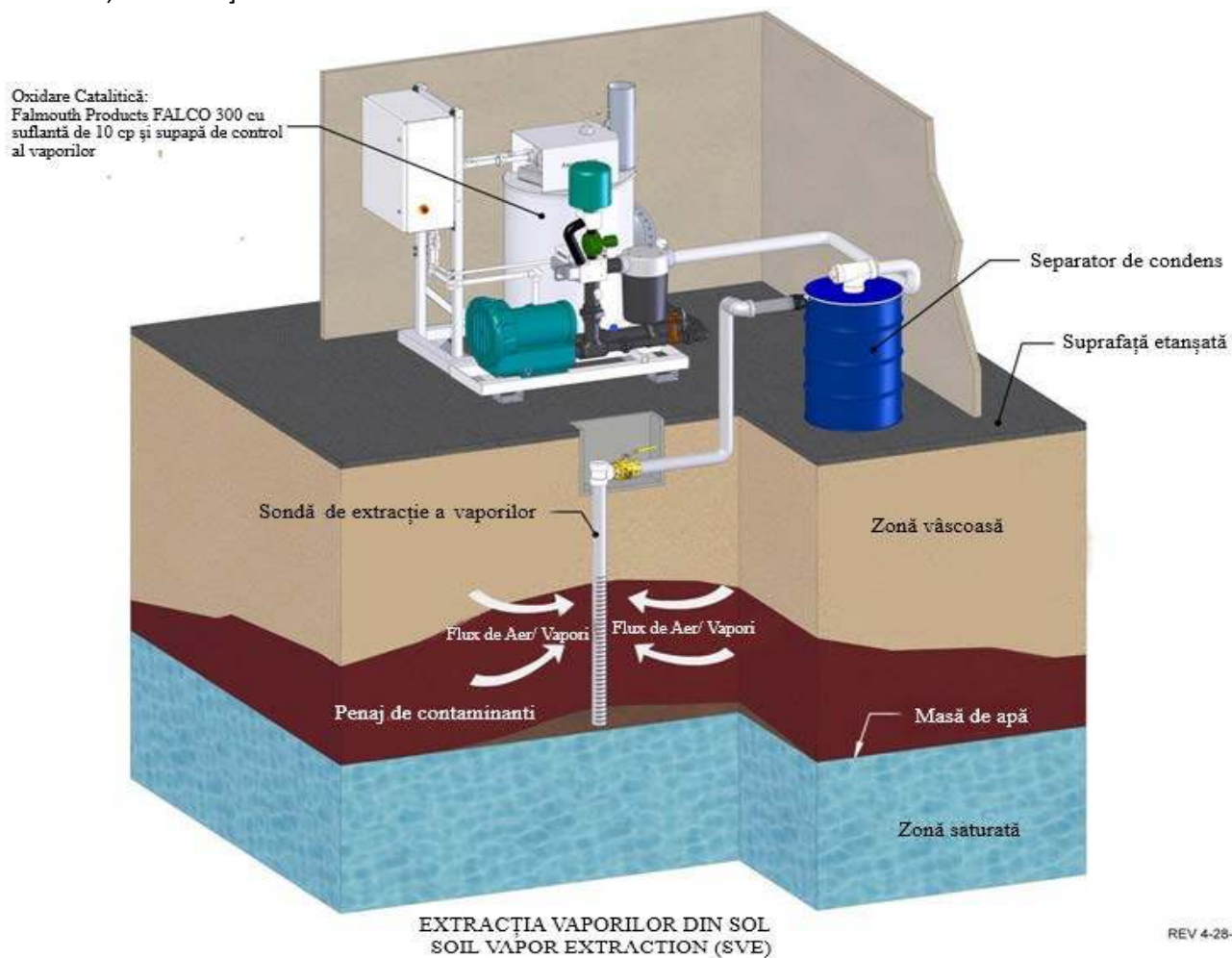
Figura 1.1- Schema SVE.
