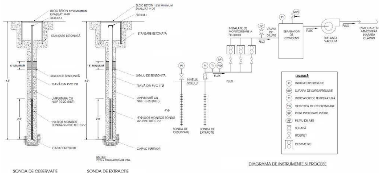
Figura 4.4- Exemplu de diagramă de proces și de instrumentație (Farallon Consulting)
